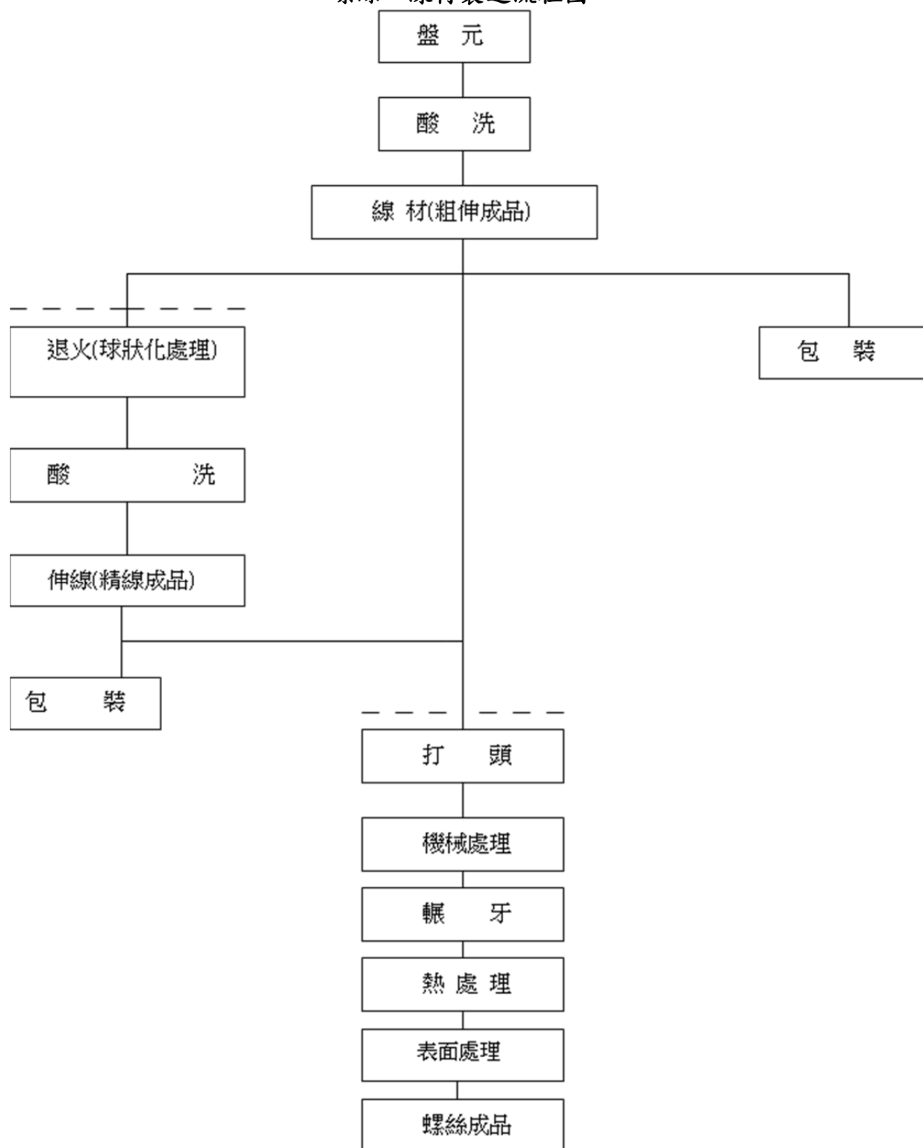
螺絲、線材製造流程圖
