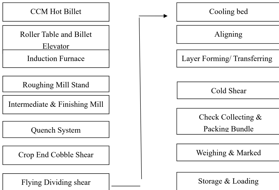
鋼筋生產流程圖
